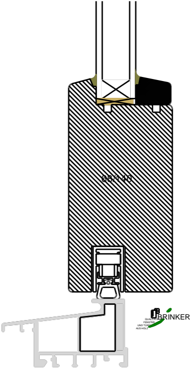
Rahmentür mit Schall - Ex
